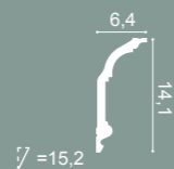
C339 | C339F 200 x 14,1 x 6,4 cm Purotouch®
