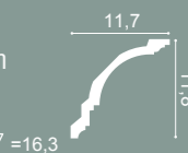
CX107 200 x 11,8 x 11,7 cm Duropolymer®
