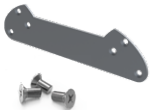
Κωδικός / Code: 4947 ΓΩΝΙΑΚΗ ΤΑΠΑ ΚΟΛΩΝΑΣ FSN-102 END CORNER CAP FOR COLUMN FSN-102
