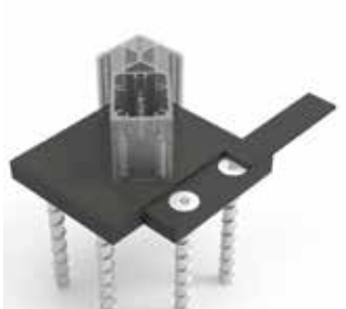
Κωδικός / Code: 4735 ΠΕΛΜΑ ΚΟΛΩΝΑΣ FSN-104 SUPPORT FOOT FOR COLUMN FSN-104
