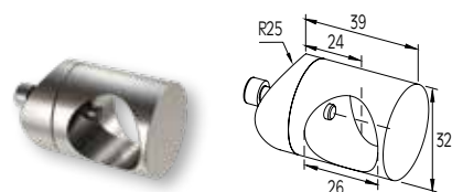
ΣΥΝΔΕΣΜΟΣ ΚΟΛΩΝΑΣ F50-101 ΜΕ ΠΡΟΦΙΛ Ø26 CONNECTOR FOR F50-101 COLUMN WITH PROFILE Ø26
