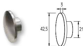
ΤΑΠΑ ΚΟΛΩΝΑΣ F50-100 END CAP FOR F50-100 COLUMN
