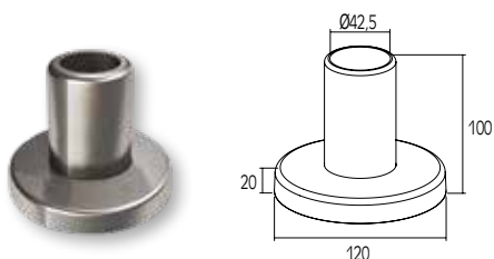
ΕΞΩΤΕΡΙΚΟ ΠΕΛΑΜ ΣΤΗΡΙΞΗΣ ΓΙΑ ΚΟΛΩΝΑ Ø42 EXTERNAL SUPPORT FOOT FOR Ø42 COLUMN
