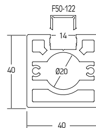
ΚΟΛΩΝΑ ΣΤΗΡΙΞΗΣ 40x40 SUPPORT COLUMN 40x40
