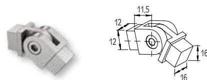
ΣΥΝΔΕΣΜΟΣ ΜΕΤΑΒΛΗΤΗΣ ΓΩΝΙΑΣ ΠΡΟΦΙΛ F50-302 ADJUSTABLE CORNER CONNECTOR FOR F50-302 PROFILE
