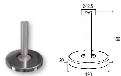
ΠΕΛΑΜ ΣΤΗΡΙΞΗΣ ΓΙΑ ΚΟΛΩΝΑ Ø42 SUPPORT FOOT FOR Ø42 COLUMN
