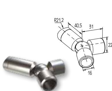
ΓΩΝΙΑΚΟΣ ΣΥΝΔΕΣΜΟΣ ΠΡΟΦΙΛ Ø16 ΜΕ ΚΟΛΩΝΑ F50-100 CONNECTOR 90° FOR PROFILE Ø16 WITH F50-100 COLUMN
