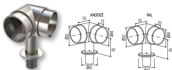
ΣΥΝΔΕΣΜΟΣ 90° ΓΙΑ ΚΟΥΠΑΣΤΗ Ø50 CONNECTOR 90° FOR HANDRAIL Ø50
