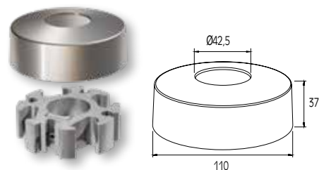
ΠΕΛΑΜ ΣΤΗΡΙΞΗΣ ΓΙΑ ΚΟΛΩΝΑ Ø42 SUPPORT FOOT FOR Ø42 COLUMN
