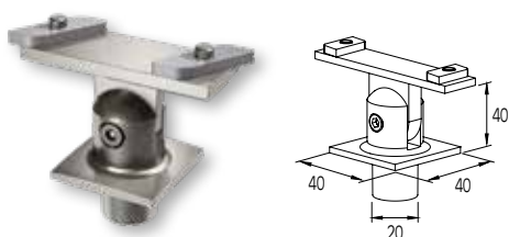
ΣΥΝΔΕΣΜΟΣ ΚΟΛΩΝΑΣ F50-102 ΜΕ ΚΟΥΠΙΑΣΤΗ F50-201 CONNECTOR FOR F50-102 COLUMN WITH F50-201 HANDRAIL
