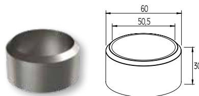
ΑΡΜΟΚΑΛΥΠΤΡΟ ΚΟΛΩΝΑΣ/ΚΟΥΠΑΣΤΗΣ F50-101 & ΚΟΥΠΑΣΤΗΣ F50-200 WALL COVER FOR F50-101 COLUMN/HANDRAIL & F50-200 HANDRAIL
