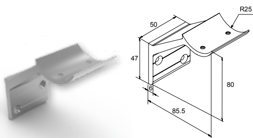
ΕΠΙΤΟΙΧΙΟ ΣΤΑΘΕΡΟ ΣΤΗΡΙΓΜΑ ΚΟΥΓΠΑΣΤΗΣ F50-200 FIXED WALL SUPPORT FOR F50-200 HANDRAIL
