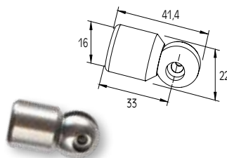
ΣΥΝΔΕΣΜΟΣ ΡΟΖΕΤΑΣ ΤΖΑΜΙΟΥ ΜΕ ΠΡΟΦΙΛ Ø16 CONNECTOR FOR GLASS ROSSETTE WITH PROFILE Ø16
