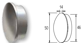
ΤΑΠΑ ΚΟΥΠΑΣΤΗΣ F50-200 END CAP FOR F50-200 HANDRAIL
