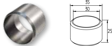
ΣΥΝΔΕΣΜΟΣ ΟΔΗΓΩΝ Ø30 ΓΙΑ ΕΥΘΕΙΑ CONNECTOR FOR GUIDE Ø30 (STRAIGHT)
