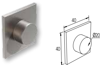
ΤΑΠΑ ΚΟΛΩΝΑΣ F50-102/109 END CAP FOR F50-102/109 COLUMN
