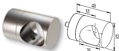
ΣΥΝΔΕΣΜΟΣ ΚΟΛΩΝΑΣ F50-102 ΜΕ ΠΡΟΦΙΛ Ø26 CONNECTOR FOR F50-102 COLUMN WITH PROFILE Ø26
