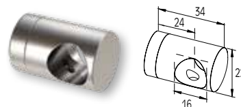
ΣΥΝΔΕΣΜΟΣ ΚΟΛΩΝΑΣ F50-102 ΜΕ ΠΡΟΦΙΛ Ø16 CONNECTOR FOR F50-102 COLUMN WITH PROFILE Ø16
