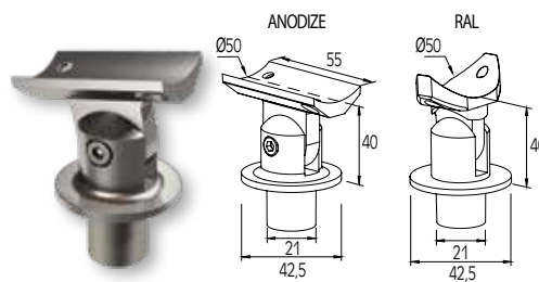
ΣΥΝΔΕΣΜΟΣ ΚΟΥΠΙΑΣΤΗΣ Ø50 ΜΕ ΚΟΛΩΝΑ Ø42 (ΣΚΑΛΑ) CONNECTOR FOR HANDRAIL Ø50 WITH COLUMN Ø42 (STAIRS)
