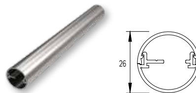
ΟΔΗΓΟΣ ΔΙΑΤΡΗΤΟΣ Ø26 PERFORATED GUIDE Ø26
