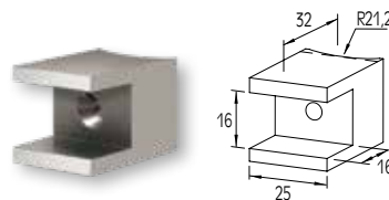
ΣΥΝΔΕΣΜΟΣ ΚΟΛΩΝΑΣ F50-100 ΜΕ ΠΡΟΦΙΛ F50-302 CONNECTOR FOR F50-100 COLUMN WITH F50-302 PROFILE
