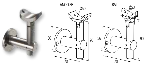
ΕΠΙΤΟΙΧΙΟ ΣΤΗΡΙΓΜΑ ΚΟΥΠΑΣΤΗΣ F50-200 WALL SUPPORT FOR F50-200 HANDRAIL
