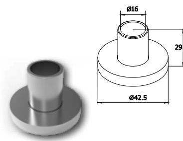
ΣΥΝΔΕΣΜΟΣ ΠΡΟΦΙΛ Ø16 mm PROFILE Ø16 mm CONNECTOR
