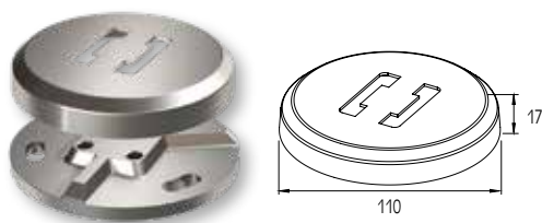
ΠΕΛΜΑ ΣΤΗΡΙΞΗΣ ΚΟΛΩΝΑΣ F50-108 SUPPORT FOOT FOR F50-108 COLUMN
