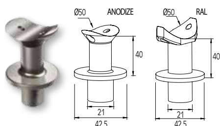
ΣΥΝΔΕΣΜΟΣ ΚΟΥΠΙΑΣΤΗΣ Ø50 ΜΕ ΚΟΛΩΝΑ Ø42 CONNECTOR FOR HANDRAIL Ø50 WITH COLUMN Ø42
