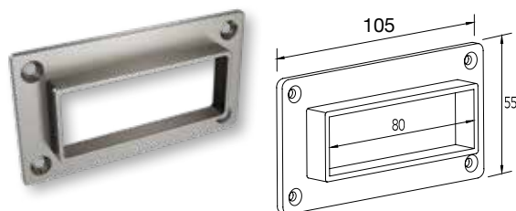
ΑΡΜΟΚΑΛΥΠΤΡΟ ΚΟΥΠΑΣΤΗΣ CLS-LINE WALL COVER FOR CLS-LINE HANDRAIL
