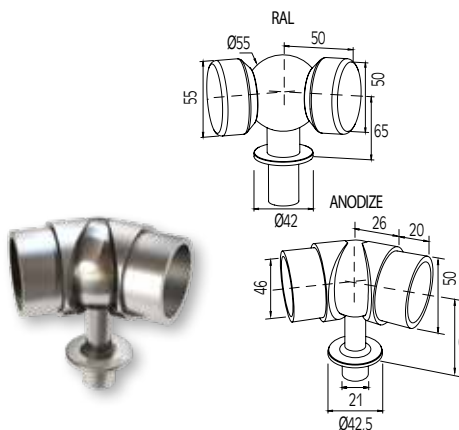
ΣΥΝΔΕΣΜΟΣ ΜΕΤΑΒΛΗΤΗΣ ΓΩΝΙΑΣ ΚΟΥΠΑΣΤΗΣ Ø50 ΜΕ ΚΟΛΩΝΑ Ø42 ADJUSTABLE CORNER CONNECTOR FOR HANDRAIL Ø50 WITH COLUMN Ø42
