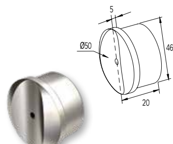
ΣΥΝΔΕΣΜΟΣ ΚΟΥΠΑΣΤΗΣ - ΚΟΥΠΑΣΤΗΣ F50-200 CONNECTOR FOR HANDRAIL WITH HANDRAIL F50-200
