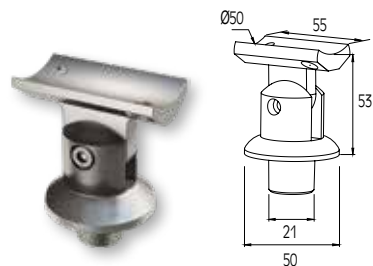
ΣΤΗΡΙΓΜΑ ΚΟΥΠΙΑΣΤΗΣ F50-200 ΜΕ ΚΟΛΩΝΑ F50-101 SUPPORT FOR HANDRAIL F50-200 WITH COLUMN F50-101
