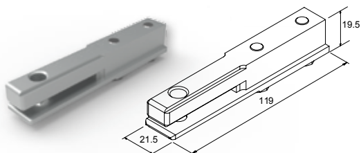
ΚΑΛΙΜΠΡΑ ΤΡΥΠΗΜΑΤΟΣ ΟΔΗΓΟΥ F50-319 HOLES CALIBRE FOR F50-319
