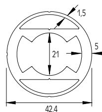
ΚΟΛΩΝΑ ΣΤΗΡΙΞΗΣ Ø42 ΕΝΙΣΧΥΜΕΝΗ SUPPORT COLUMN Ø42 (HEAVY-DUTY)
