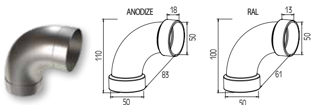
ΓΩΝΙΑΚΟΣ ΣΥΝΔΕΣΜΟΣ 90° ΚΟΥΠΑΣΤΩΝ Ø50 CONNECTOR 90° FOR HANDRAIL Ø50
