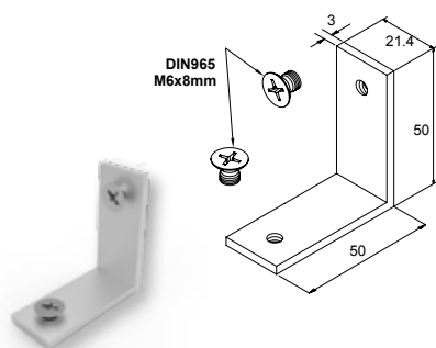
ΓΩΝΙΑ ΣΥΝΔΕΣΗΣ ΟΔΗΓΟΥ F50-319 CONNECTOR FOR F50-319 GUIDE
