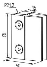
ΣΤΗΡΙΓΜΑ ΤΖΑΜΙΟΥ 8-10 mm GLASS SUPPORT 8-10mm
