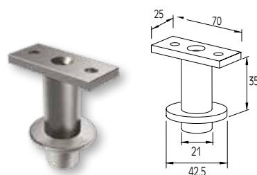
ΣΥΝΔΕΣΜΟΣ ΚΟΛΩΝΑΣ F50-100 ΜΕ ΚΟΥΠΙΑΣΤΗ F50-201 CONNECTOR FOR F50-100 COLUMN WITH F50-201 HANDRAIL
