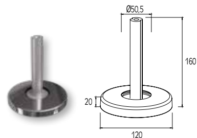
ΠΕΛΑΜ ΣΤΗΡΙΞΗΣ ΓΙΑ ΚΟΛΩΝΑ Ø50 SUPPORT FOOT FOR Ø50 COLUMN
