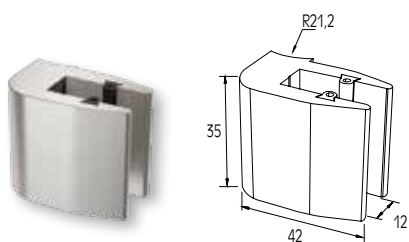
ΣΤΗΡΙΓΜΑ ΤΖΑΜΙΟΥ 8-10mm ΜΟΝΟ ΓΙΑ ΚΟΛΩΝΑ F50-103 SINGLE GLASS SUPPORT 8-10mm FOR F50-103 COLUMN
