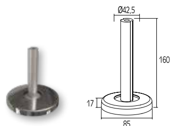
ΠΕΛΑΜ ΣΤΗΡΙΞΗΣ ΓΙΑ ΚΟΛΩΝΑ Ø42 SUPPORT FOOT FOR Ø42 COLUMN
