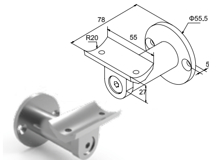
ΕΠΙΤΟΙΧΙΟ ΣΤΗΡΙΓΜΑ ΚΟΥΠΑΣΤΗΣ Ø40 WALL SUPPORT FOR Ø40 HANDRAIL
