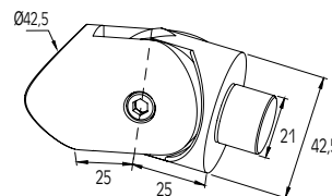
ΣΥΝΔΕΣΜΟΣ ΚΟΛΩΝΑΣ ΜΕ ΚΟΛΩΝΑ F50-100 (ΣΚΑΛΑ) CONNECTOR FOR COLUMN WITH COLUMN F50-100 (STAIRS)
