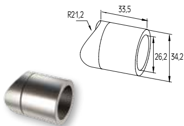
ΣΥΝΔΕΣΜΟΣ ΚΟΛΩΝΑΣ F50-100 ΜΕ ΠΡΟΦΙΛ Ø26 CONNECTOR FOR F50-100 COLUMN WITH PROFILE Ø26
