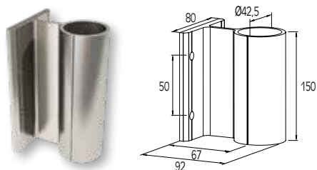
ΕΞΩΤΕΡΙΚΟ ΕΠΙΤΟΙΧΙΟ ΣΤΗΡΙΓΜΑ ΓΙΑ ΚΟΛΩΝΑ Ø42 EXTERNAL WALL SUPPORT FOR COLUMN Ø42
