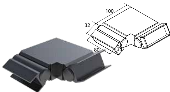
ΣΥΝΔΕΣΜΟΣ 90° ΜΕΤΑΒΛΗΤΗΣ ΓΩΝΙΑΣ ΚΟΥΠΙΑΣΤΗΣ CLS-202 (ΣΚΑΛΑ) ADJUSTABLE CORNER CONNECTOR 90° FOR CLS-202 HANDRAIL (STAIRS)
