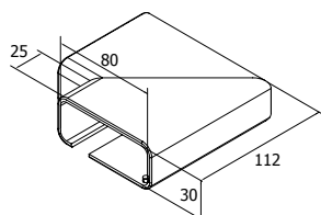
ΣΥΝΔΕΣΜΟΣ ΚΟΥΠΙΑΣΤΩΝ (ΕΣΩΤΕΡΙΚΟΣ) F50-203/223 ΓΩΝΙΑ ΜΕ ΥΠΟΔΟΧΗ ΤΖΑΜΙΟΥ CONNECTOR (INSIDE CORNER) FOR F50-203/223 HANDRAIL WITH GLASS PANEL SLIT
