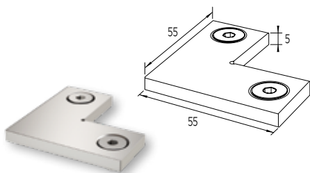
ΣΥΝΔΕΣΜΟΣ 90° ΓΙΑ ΚΟΥΠΑΣΤΗ CLS-202 CONNECTOR 90° FOR CLS-202 HANDRAIL
