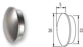
ΤΑΠΑ ΓΙΑ ΠΡΟΦΙΛ F50-304 END CAP FOR F50-304 PROFILE
