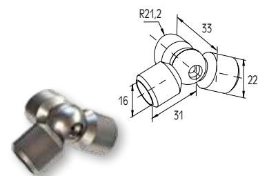
ΣΥΝΔΕΣΜΟΣ ΜΕΤΑΒΛΗΤΗΣ ΓΩΝΙΑΣ ΠΡΟΦΙΛ Ø16 ΜΕ ΚΟΛΩΝΑ F50-100 ADJUSTABLE CORNER CONNECTOR FOR PROFILE Ø16 WITH F50-100 COLUMN
