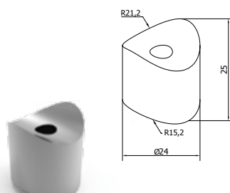
ΣΥΝΔΕΣΜΟΣ F50-307/327 ΜΕ ΚΟΛΩΝΑ F50-103/123 CONNECTOR FOR F50-307-327 WITH F50-103/123 COLUMN
