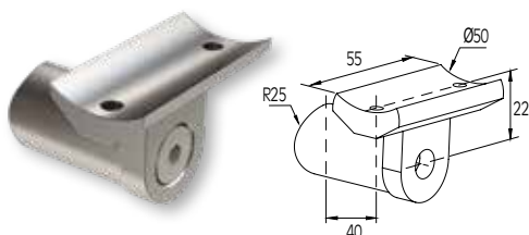
ΕΞΩΤΕΡΙΚΟ ΣΤΗΡΙΓΜΑ ΚΟΥΠΙΑΣΤΗΣ F50-200 ΜΕ ΚΟΛΩΝΑ F50-101 EXTERNAL SUPPORT FOR HANDRAIL F50-200 WITH COLUMN F50-101
