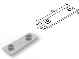
ΕΥΘΕΙΑ ΣΥΝΔΕΣΗΣ ΟΔΗΓΟΥ F50-319 LINEAR CONNECTOR FOR F50-319 GUIDE
