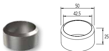
ΑΡΜΟΚΑΛΥΠΤΡΟ ΚΟΛΩΝΑΣ Ø42 COVER FOR COLUMN Ø42
