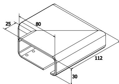
ΣΥΝΔΕΣΜΟΣ 90° ΚΟΥΠΙΑΣΤΩΝ F50-203/223 CONNECTOR 90° F50-203/223 HANDRAIL
