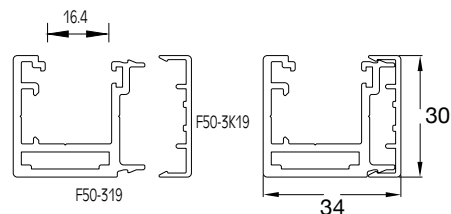
ΚΑΠΑΚΙ ΟΔΗΓΟΥ F50-319 COVER FOR F50-319 GUIDE
