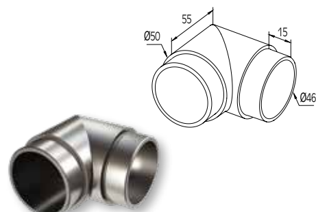
ΣΥΝΔΕΣΜΟΣ 90° ΓΙΑ ΚΟΥΠΑΣΤΗ Ø50 CONNECTOR 90° FOR HANDRAIL Ø50
