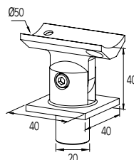
ΣΤΗΡΙΓΜΑ ΚΟΥΠΑΣΤΗΣ F50-200 ΜΕ ΚΟΛΩΝΑ F50-102 (ΣΚΑΛΑ) SUPPORT FOR F50-200 HANDRAIL WITH F50-102 COLUMN (STAIRS)
