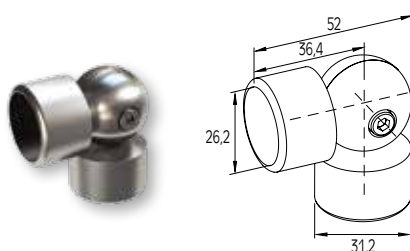
ΣΥΝΔΕΣΜΟΣ ΜΕΤΑΒΛΗΤΗΣ ΓΩΝΙΑΣ ΠΡΟΦΙΛ Ø26 ADJUSTABLE CORNER CONNECTOR FOR PROFILE Ø26
