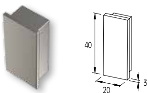
ΤΑΠΑ ΓΙΑ ΠΡΟΦΙΛ 59-009 (40x20) END CAP FOR PROFILE 59-009 (40x20)
