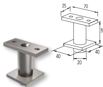
ΣΤΗΡΙΓΜΑ ΚΟΛΩΝΑΣ F50-102 ΜΕ ΚΟΥΠΑΣΤΗ F50-201 SUPPORT FOR F50-102 COLUMN WITH F50-201 HANDRAIL
