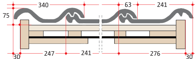
Maße Doppelkremper
